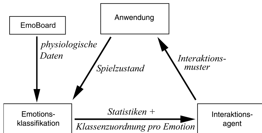
Abbildung 5.6: Schematische Darstellung der einzelnen Komponenten und der Fluss der Daten zwischen ihnen
