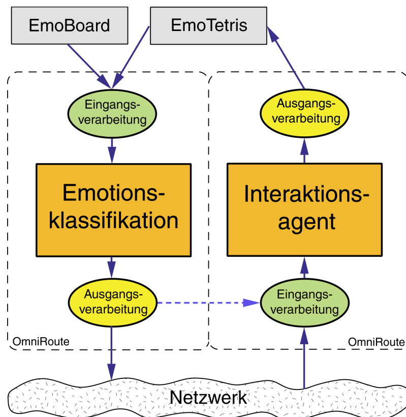
Abbildung 4.9: Schematischer Aufbau des EmoControl-Frameworks mit seinen Komponenten und der Verarbeitungsabfolge: OmniRoute synchronisiert die Daten und leitet sie weiter
