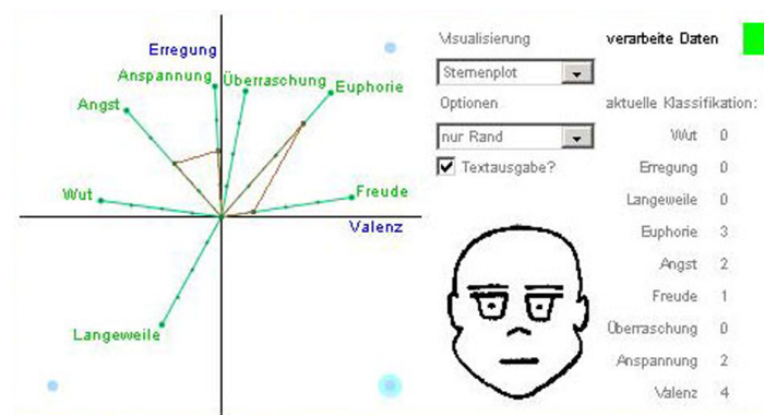
Abbildung 4.6: Komplettierte Visualisierung mit mehreren redundanten Möglichkeiten, den geschätzten emotionalen Zustand des Spielers abzulesen
