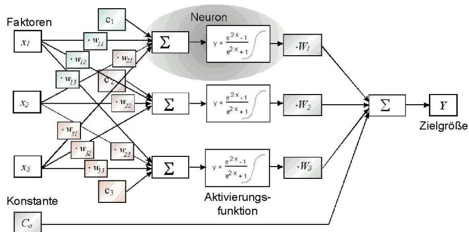
Abbildung 3.2: Prinzipieller Aufbau eines Neuronalen Netzes
