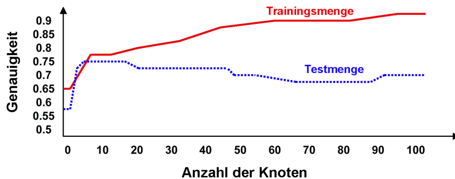
Abbildung 3.1: Bei zunehmender Komplexität passt das erlernte Netz immer besser zu den Trainingsdaten, wird aber gleichzeitig schlechter bei der Vorhersage unbekannter Testdaten: es ist überangepasst (engl. overfitting ).
