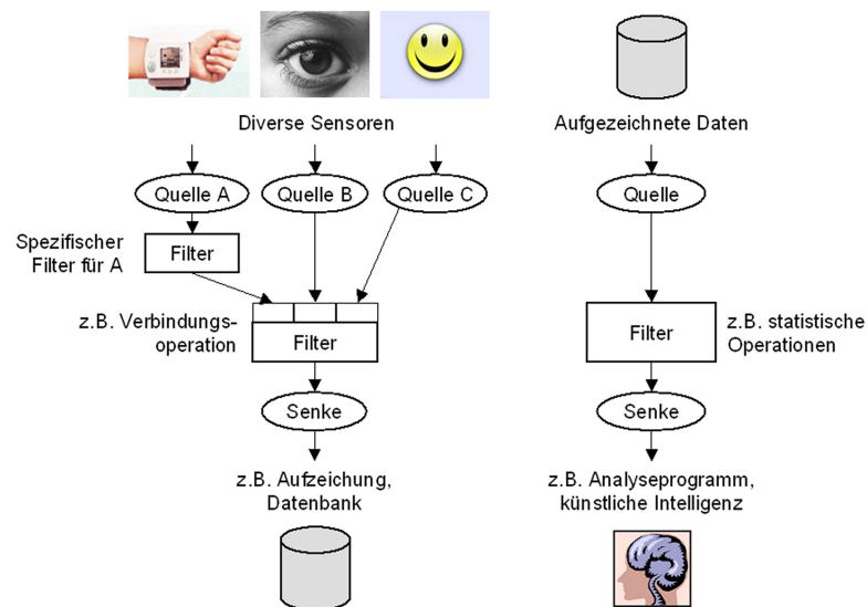
Abbildung 5: Zwei Beispiele der Ereignisverarbeitung in OmniRoute mit Quellen, Filter und Senken: Links aus unterschiedlichen Sensoren gespeist ( online Verarbeitung), rechts aus einer Sitzungsaufnahme ( offline Verarbeitung) (aus Mader 2004)
