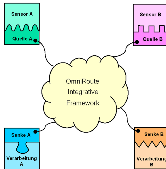
Abbildung 4.7: OmniRoute als Framework hinter EmoControl: Synchronisation und Weiterleiten der Daten (Darstellung angelehnt an Mader 2004)
