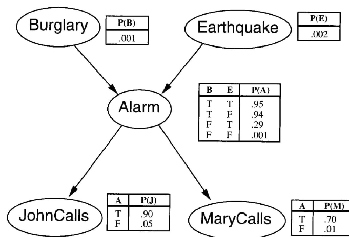
Abbildung 3.4: Beispiel eines einfachen Bayesschen Netzwerks (aus Russell u. Norvig (1995))
