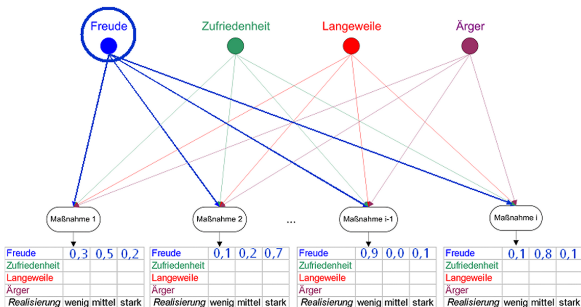
Abbildung 5.5: Schematische Darstellung der Funktionsweise bei der Abfrage Bayesscher Netze
