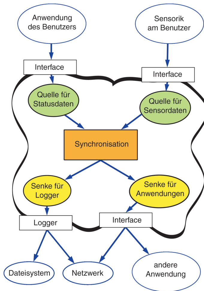
Abbildung 5.1: Synchronisation der physiologischen Daten von der Sensorik und der Statusdaten der Anwendung
