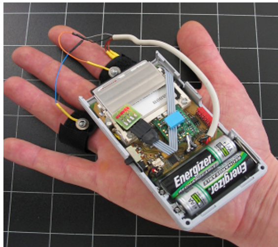
Abbildung 4.5: Sensorik und Steuergerät zur Erfassung der physiologischen Größen Puls, Hautwiderstand und Hauttemperatur
